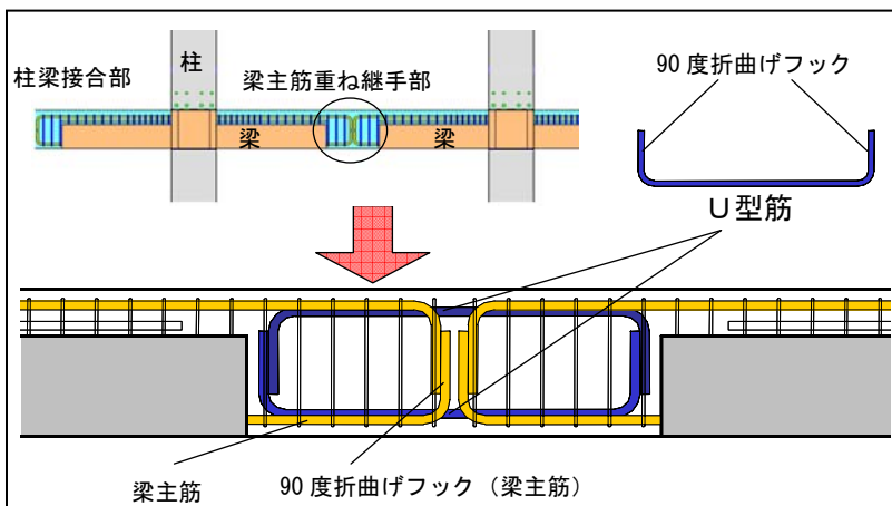
『戸田式RC梁重ね継手法』工法概念図
