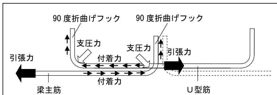
梁主筋間の引張力伝達の概念図
