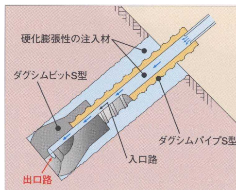
図-1 同時削孔注入の仕組み
