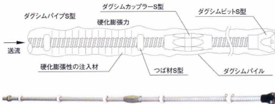
図-2 芯材構造図
