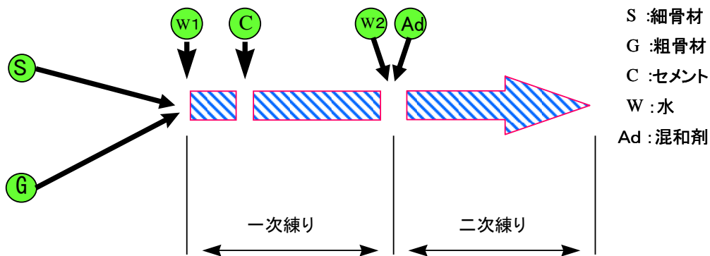
図-1 SECコンクリートの製造フロー
