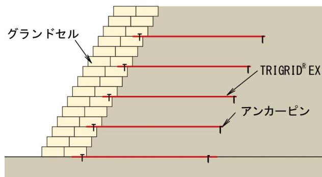
(b) コンクリートブロック式補強土壁
