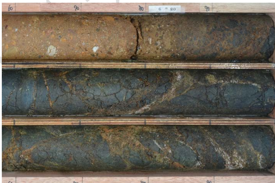
写真 10-12 洗浄してマッドケーキを取り除いた状態
