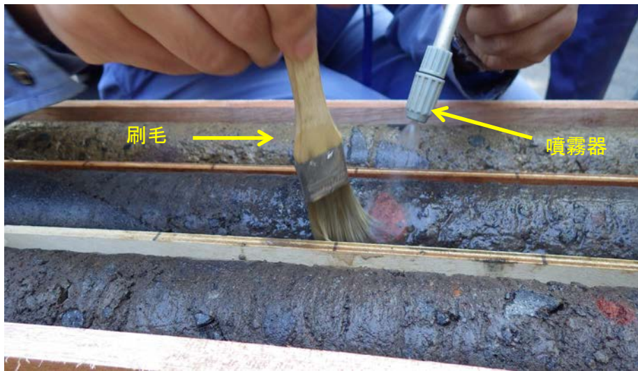
写真 10-10 噴霧器と刷毛を使った洗浄
